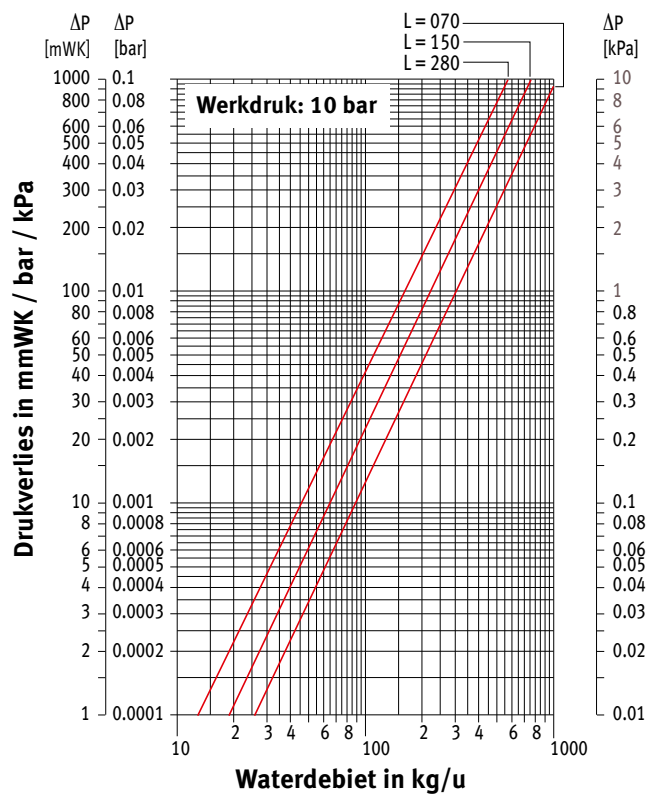
DRUKVERLIES TYPE 11
