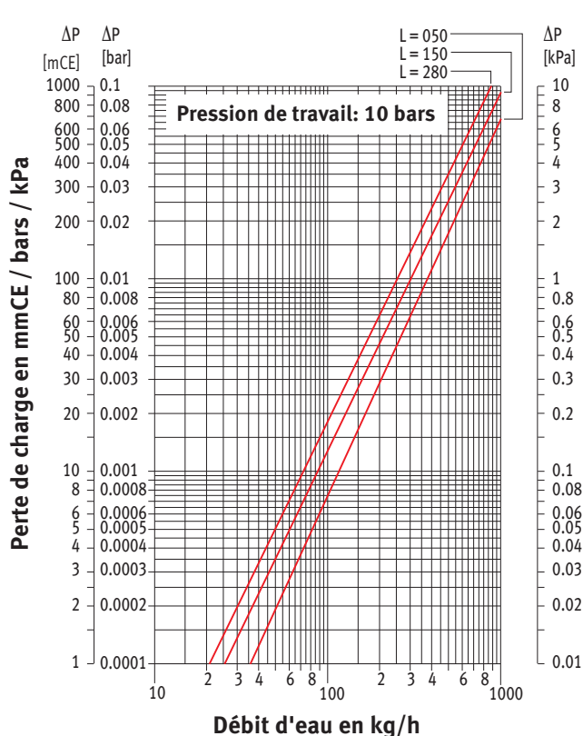
PERTE DE CHARGE TYPE 16
